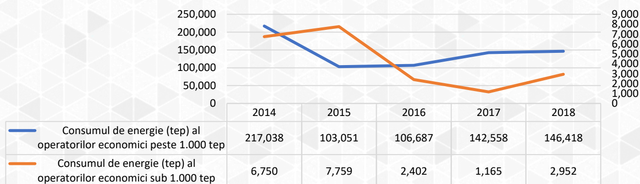
Figura 43 Evoluția consumului de energie pe tipuri de operatori, județul Dolj
