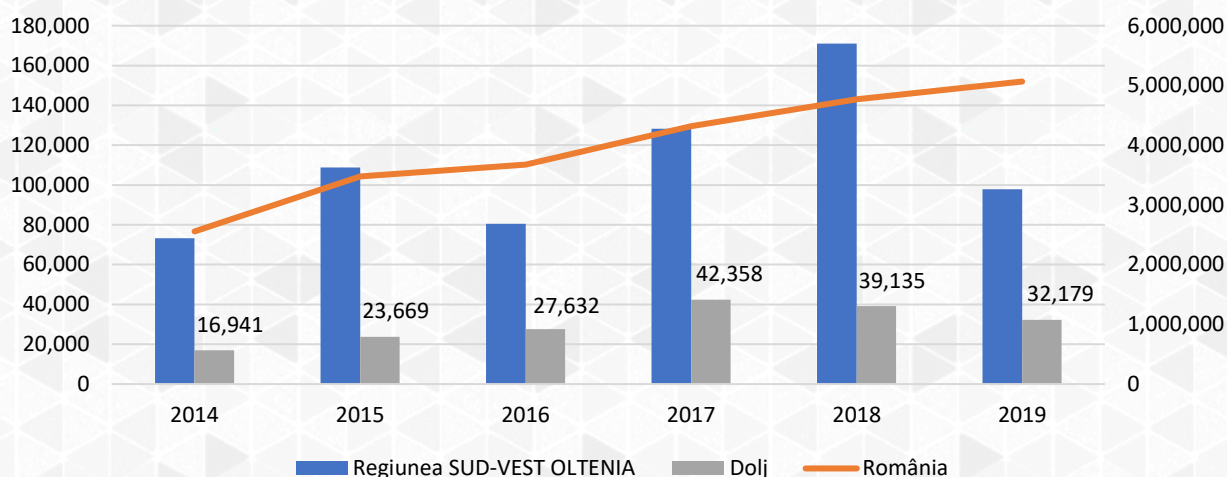
Figura 103 Evoluția cheltuielilor totale din activitatea de cercetare-dezvoltare la nivel județean, regional și național (mii lei), în perioada 2014-2019
