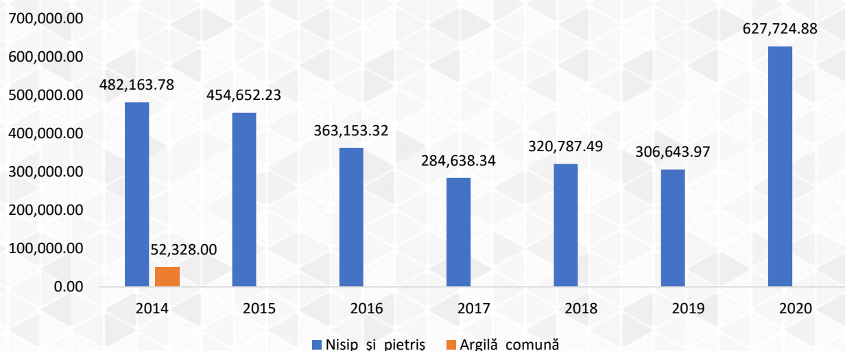
Figura 16 Cantități de resurse minerale extrase în perioada 2014-2020 pe teritoriul județului Dolj
