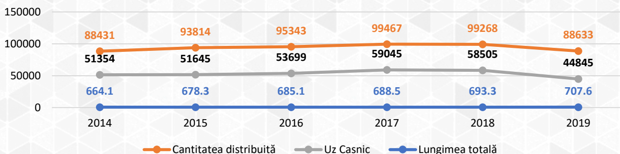
Figura 36 Evoluția lungimii conductelor de distribuție a gazelor naturale și a cantității de gaze naturale distribuite din județ, în perioada 2014-2019
