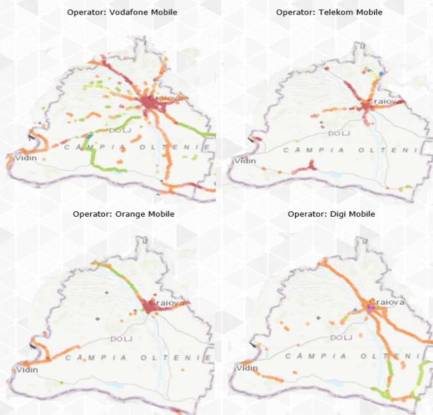
Figura 48 Hartă acoperire 3G, 4G, 5G din județul Dolj
