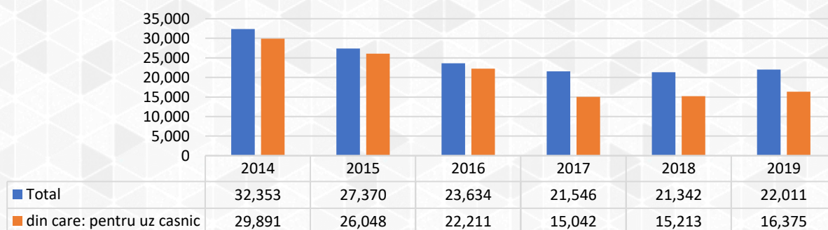
Figura 32 Evoluția cantității totale de apă potabilă distribuită consumatorilor în județul Dolj (mii m 3 ), în perioada 2014-2019
